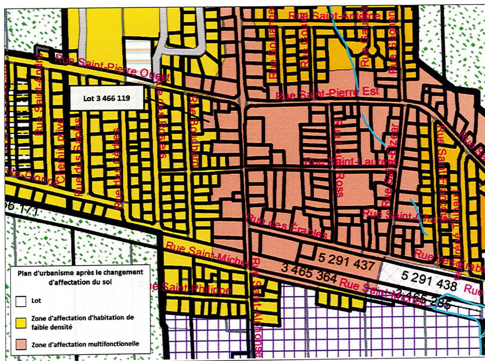
Plan 2 : Plan des grandes affectations du sol après la modification
